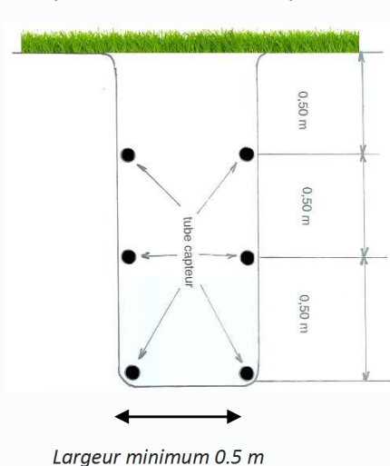
Coupe tranchée avec 3 capteurs
