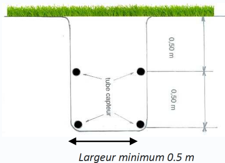
Coupe tranchée avec 2 capteurs
