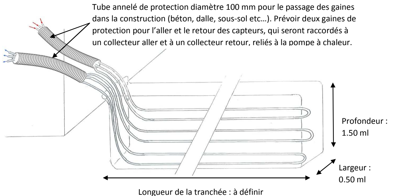
Coupe tranchée avec 2 capteurs
